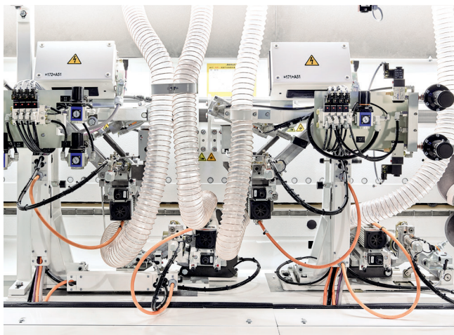
跟踪装置：独立的4马达同步绕转加工，达到完美的修圆角效果。
