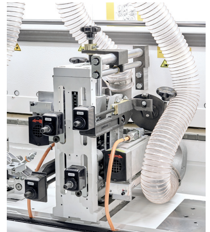
斜角/圆弧精修装置： 手动调节斜角和圆弧加工。
