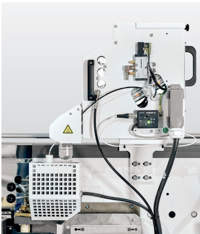
涂胶和预熔装置： 及时提供胶水，完美的涂胶效果。根据实际需要熔化胶水，持续供应新鲜的胶水。
