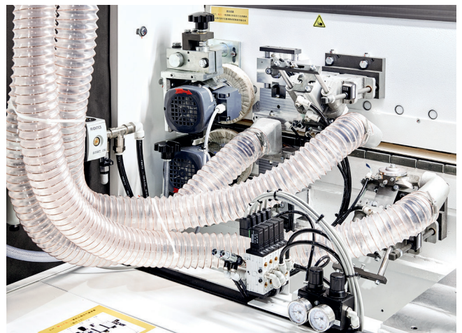
完美的修整单元：仿形刮刀装置可使封边带边部更光滑，平刮刀装置清除残留的胶水，抛光装置清洁表面，从而提高工件的质量。
